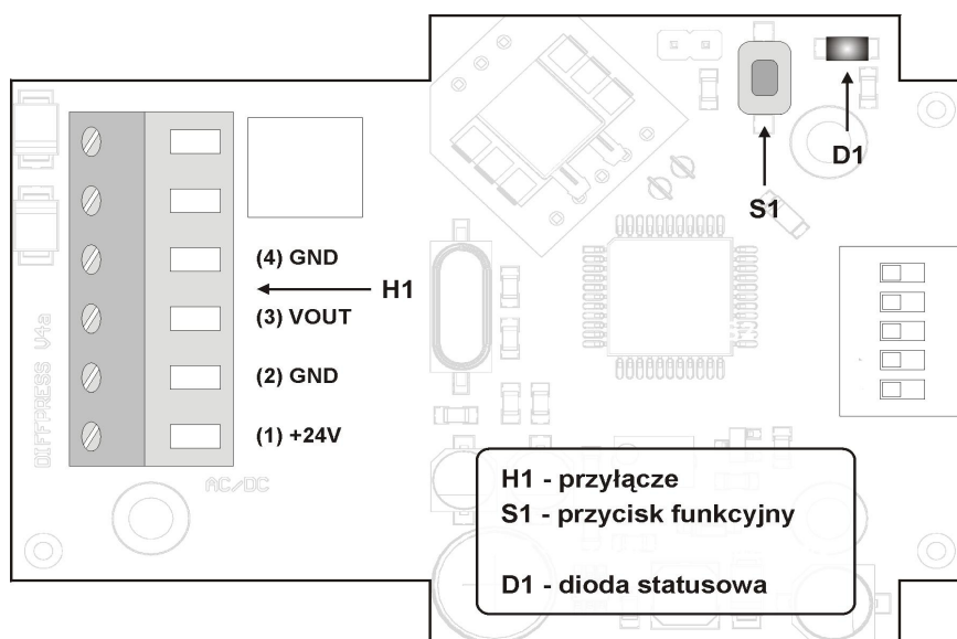
Rysunek 2. Opis wyprowadzeń przetwornika.
